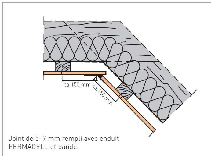
Figure 17 : 1. Joint classique avec bande
