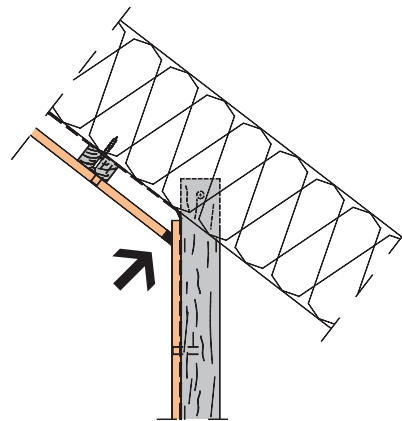
Raccord horizontal plafond rampant
