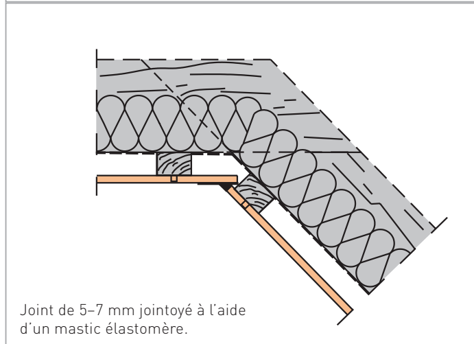
Figure 19 : 3. Joint à élasticité permanente (par exemple enduit acrylique, mastic élastomère)
