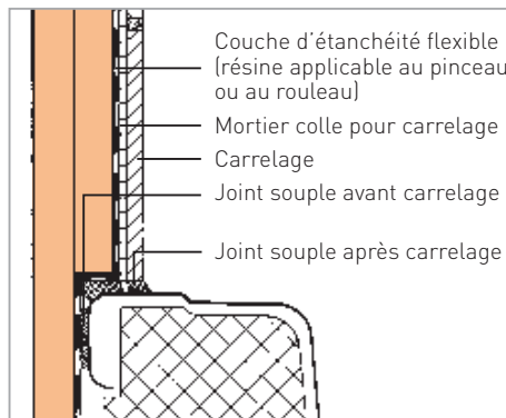
Figure 28 : Même chose avec pose d'une deuxième peau au dessus de l'appareil receur.
