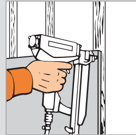
Figure 10 : Agrafage sur ossature bois
