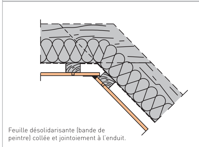
Figure 18 : 2. Jointoyement avec feuille désolidarisante
