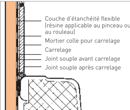
Figure 27 : Raccord horizontal d'une cloison simple peau avec un appareil receur (douche, baignoire).
